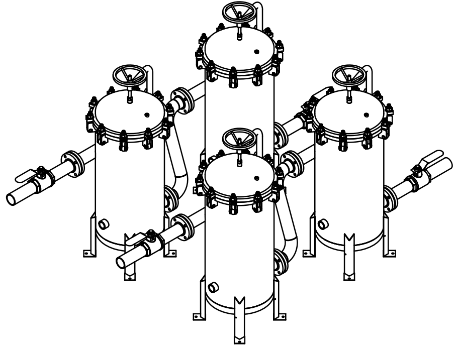
ИЗОМЕТРИЧЕСКИЙ ВИД
